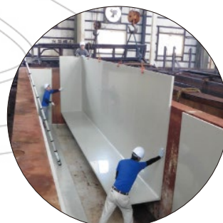
PPパネルタンク 製作実績
