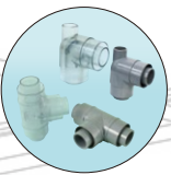
実管と保護管を スベーサーで一体化 塩ビ製 二重管継手 (成形品)
