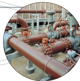
硬質塩化ビニルライニング鋼管・継手 施工現場
