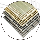
FRP製 歩道用 ファイバークレーチング (R-6) 25×100メッシュタイプ
